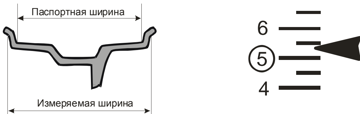
а – паспортная и измеряемая ширина диска б – ближайшее меньшее значение 5 дюймов.
